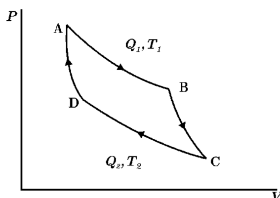
Рис. 2. Цикл Карно
