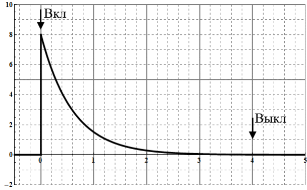
Рис. 9. Зависимость тока, текущего через амперметр, от времени
