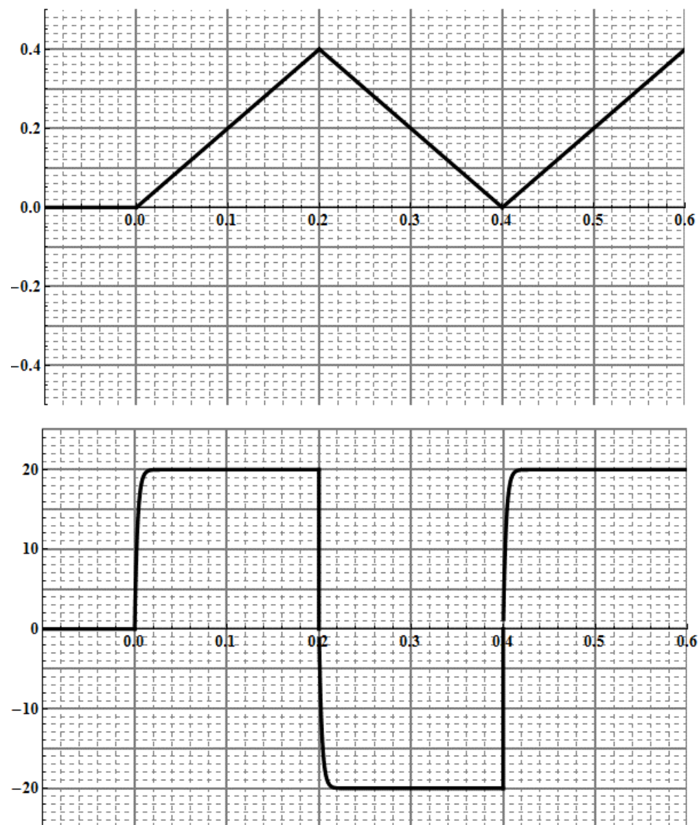
Рис. 7. Треугольный сигнал U и сигнал амперметра I
