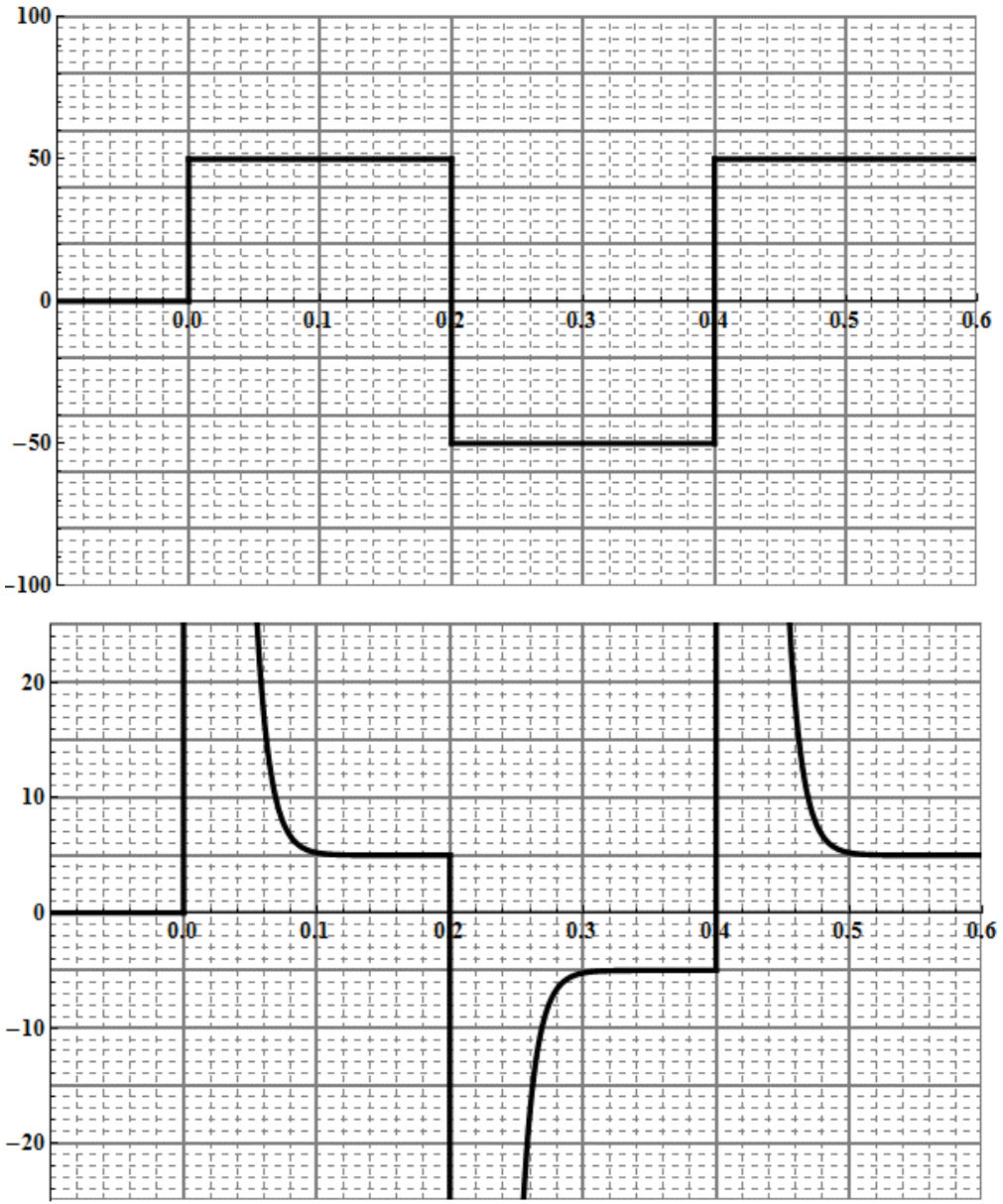
Рис. 6. Прямоугольный сигнал U и сигнал амперметра I
