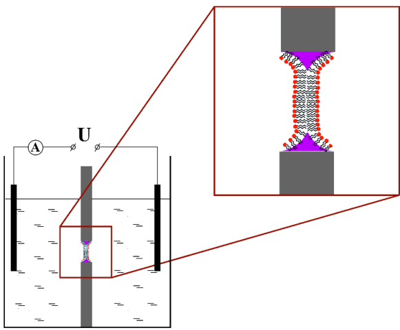
Рис. 5. Схема установки, содержащей черную липидную мембрану
