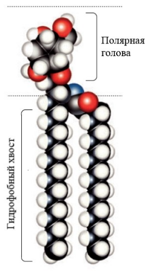
Рис.1. Молекула липида
