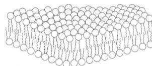
Рис.2. Липидный бислой
